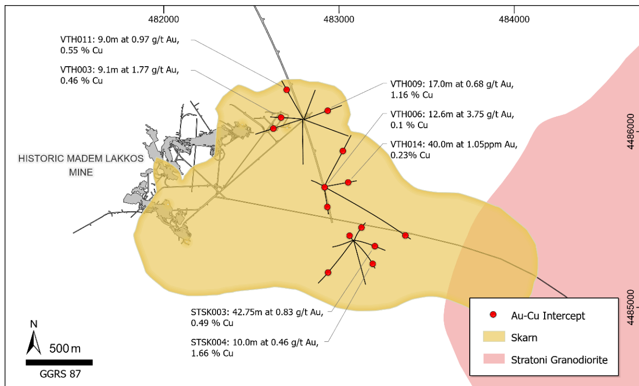
Εικόνα 9: Χάρτης του κοιτάσματος χρυσού-χαλκού Σκαρν Στρατωνίου με επισήμανση γεωτρήσεων με αξιοσημείωτα γεωχημικά αποτελέσματα.
